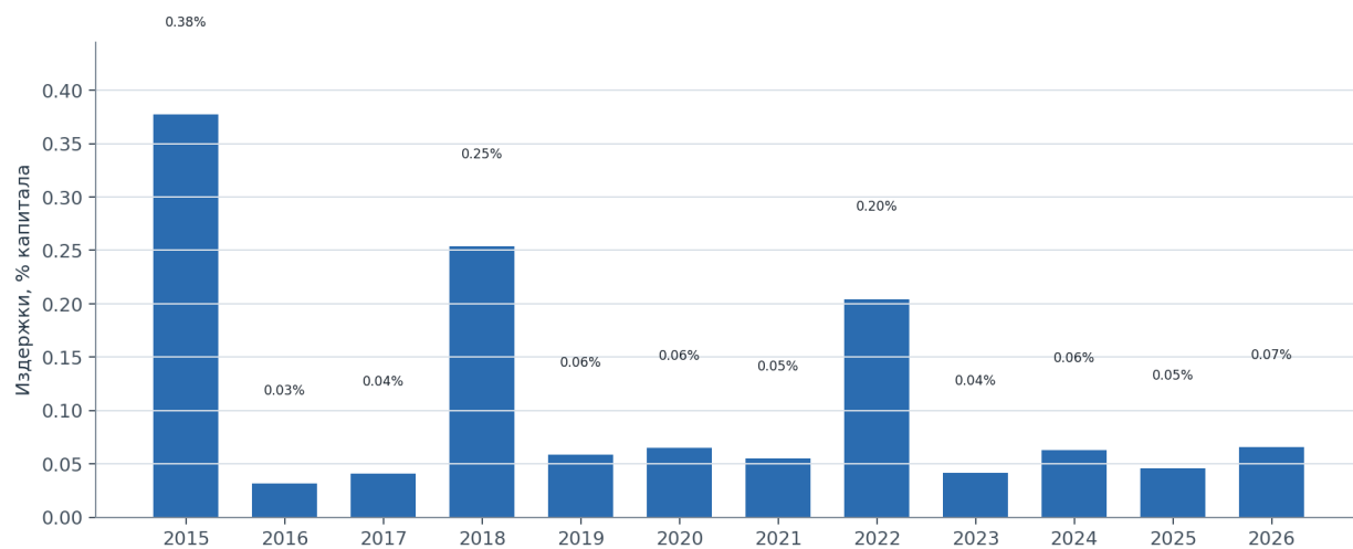
Рисунок 2. Комиссии и проскальзывание как доля капитала на каждой ребалансировке.
